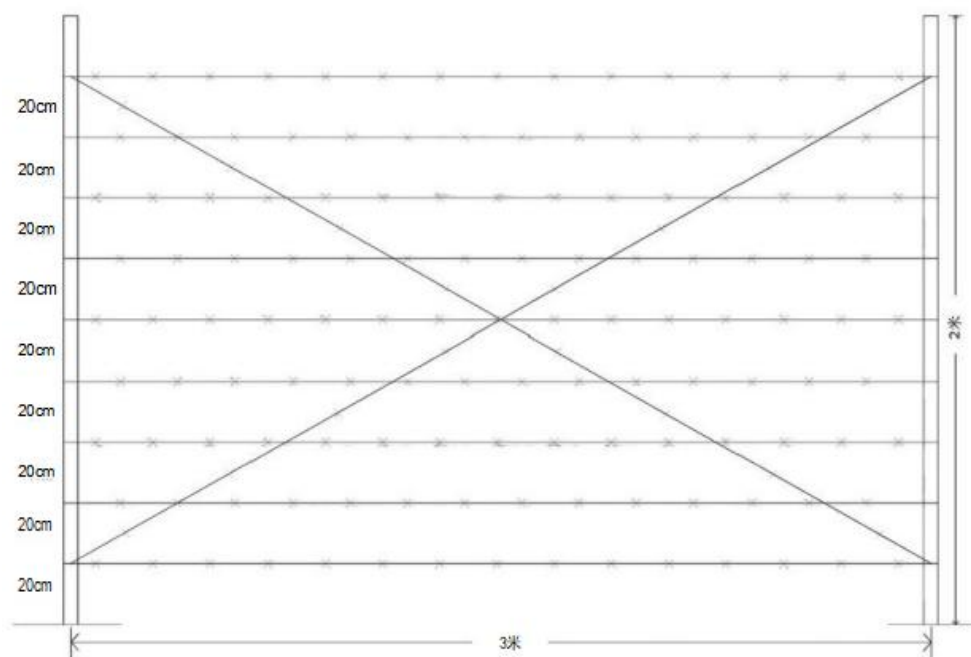
图4-1 围栏安装示意图
