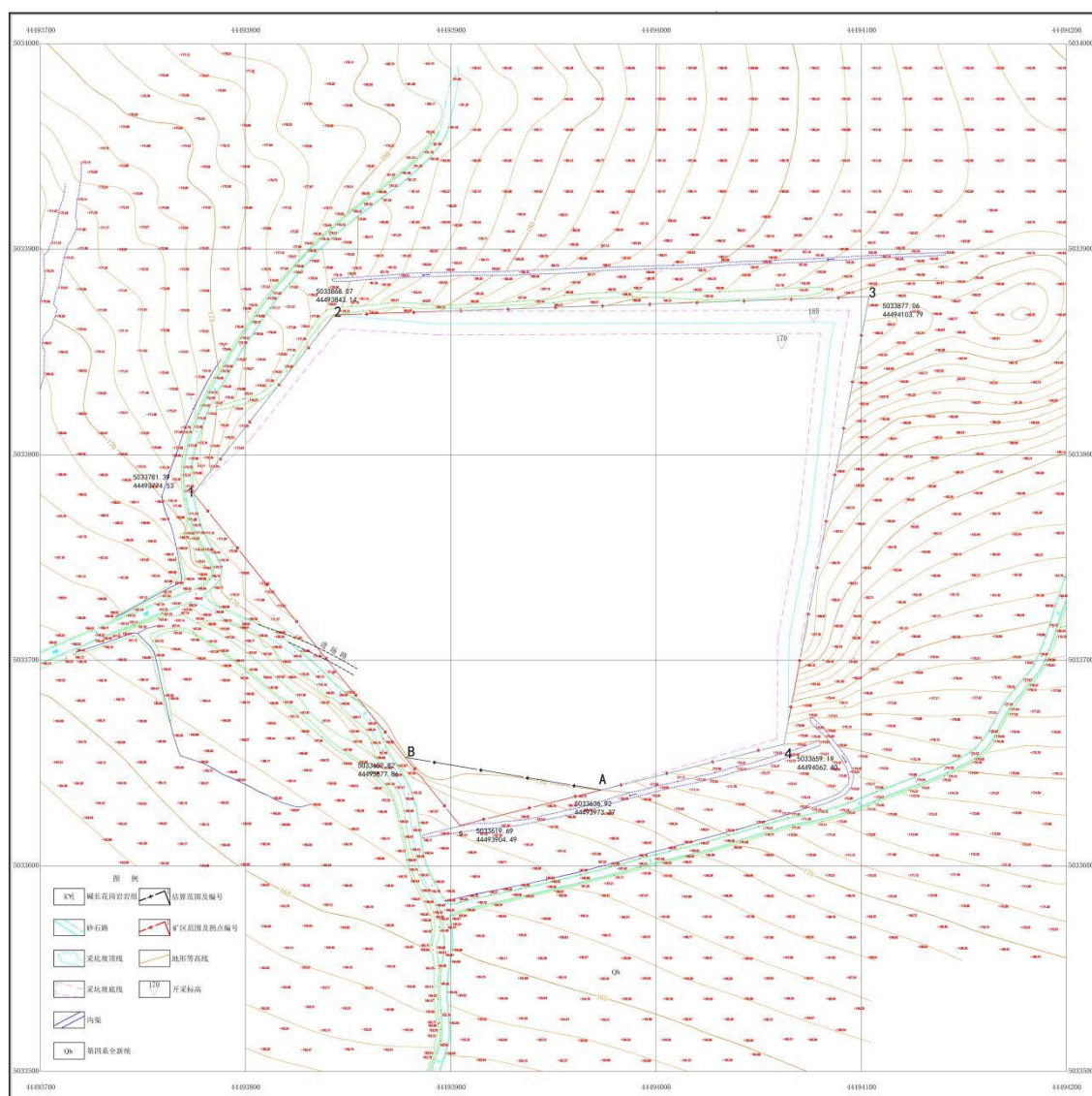
图1-3 露天开采境界图
