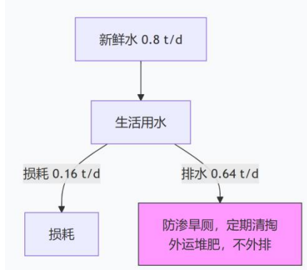
图 2-1 本项目水量平衡图（t/d）
