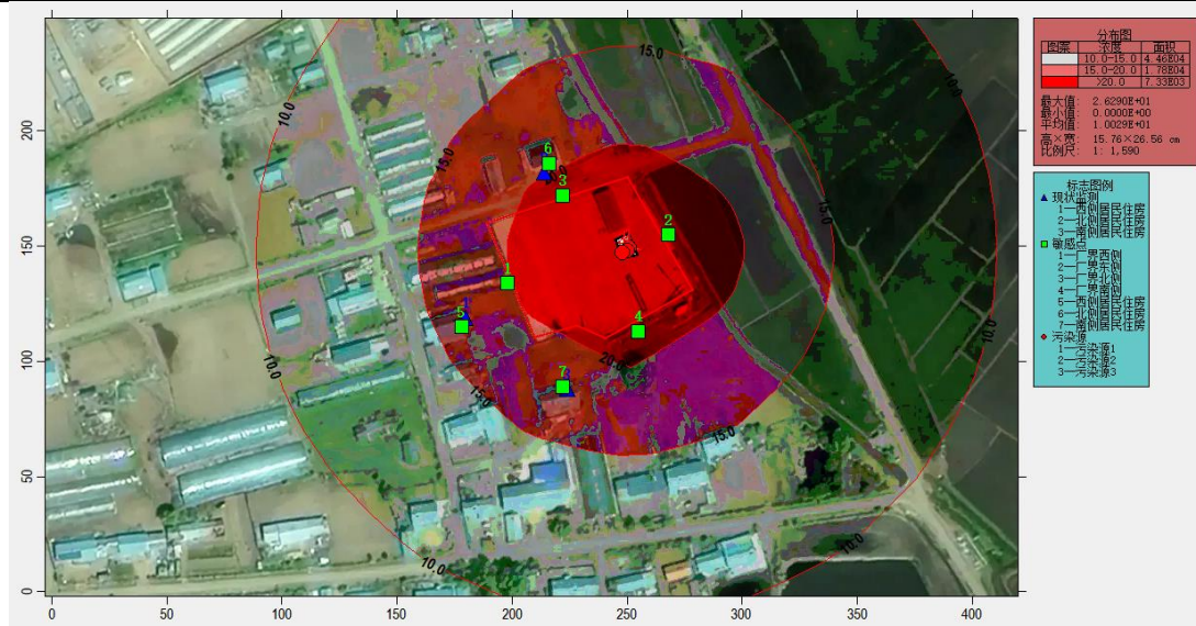
图 4-1 厂界噪声及敏感点预测图
