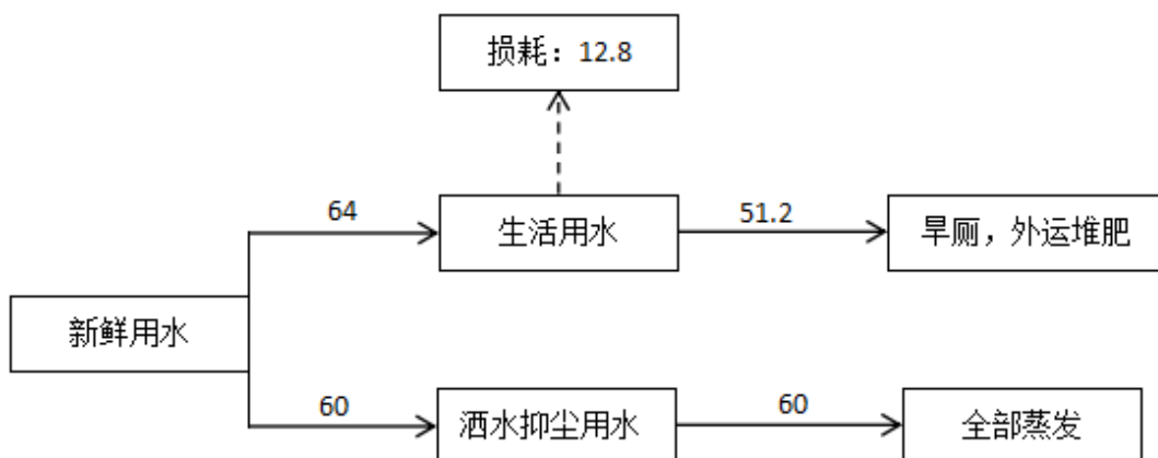
图 2-1 本项目水量平衡图 (单位: t/a)
